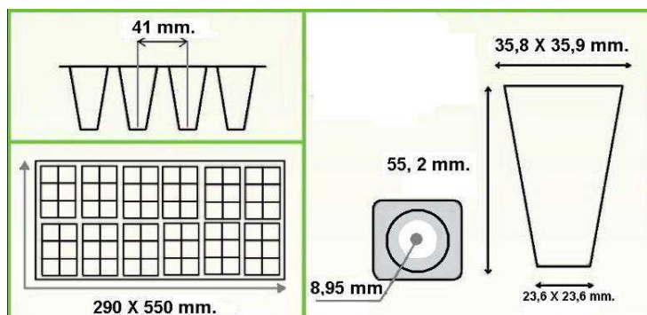
Dimensiones bandeja de 72 cavidades (6X12)
